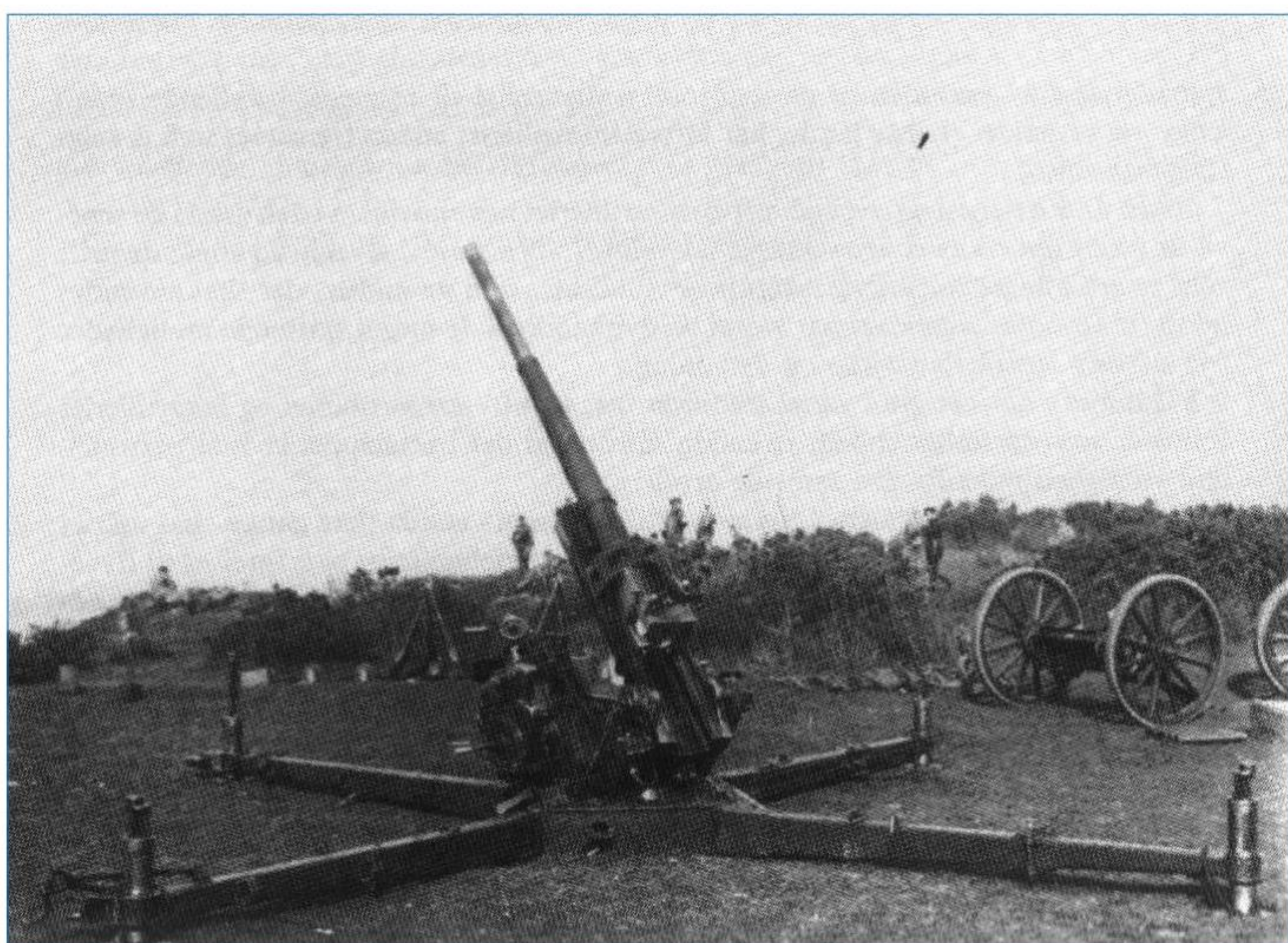
75 mm Luftværnskanon 1932
