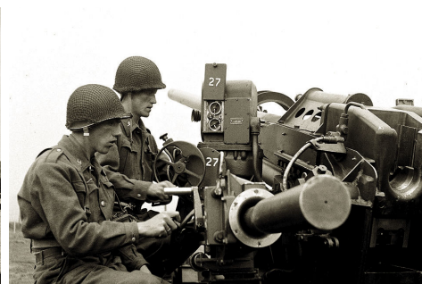
90 mm Luftværnskanon M/50
