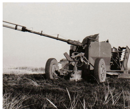
40 mm Luftværnskanon, L70
